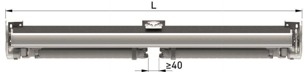
L para máquina por dentro ó motor L for gear inside or motor L pour treuil par dedans ou moteur L per arganello interiore o motore
