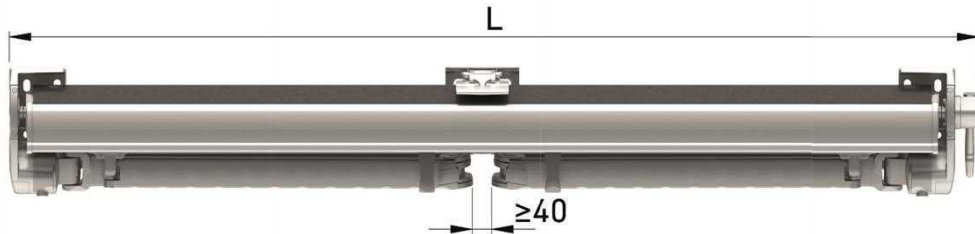
L para máquina por fuera con suplemento 80081660 L for gear outside with supplement 80081660 L pour treuil dehors avec supplément 80081660 L per arganello esteriore con supplemento 80081660
