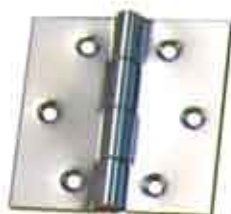
Bisagra fija de 70x70 en doble chapa galvanizada de 1,2 mm
